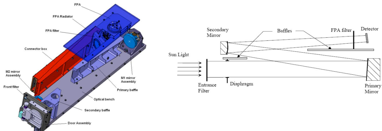
Figuur 29: De opbouw van de SWAP UV telescoop
