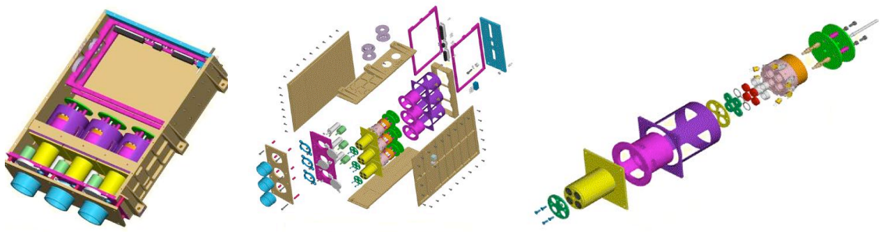
Figuur 27: De LYRA radiometer, steeds verder gedemonteerd
